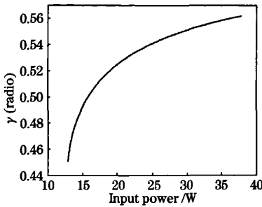
图5 激光器稳定单频工作的条件,最小 \gamma 值与抽运功率的关系
