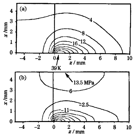
图2 端面抽运键合晶体中的温度(a)和应力(b)分布 Fig. 2 Temperature (a) and stress (b) distributions for the composite crystal
