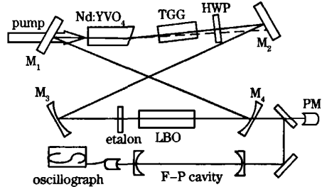
图6 楔形Nd:YVO 4 晶体激光器实验装置
