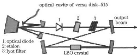
图 4 薄片式激光器实验装置
