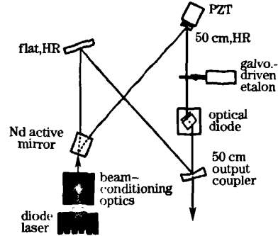
图 9 标准具辅助调谐激光器 Fig. 9 Broadband tuning laser by using etalon
