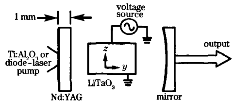
图7 电光效应调谐激光器实验装置
