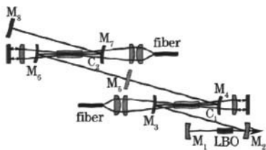
图 3 采用低吸收晶体的激光器装置
